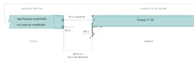
Reforç estructural de voladiu
