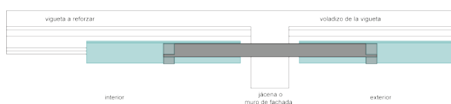
Substitució funcional de voladiu
